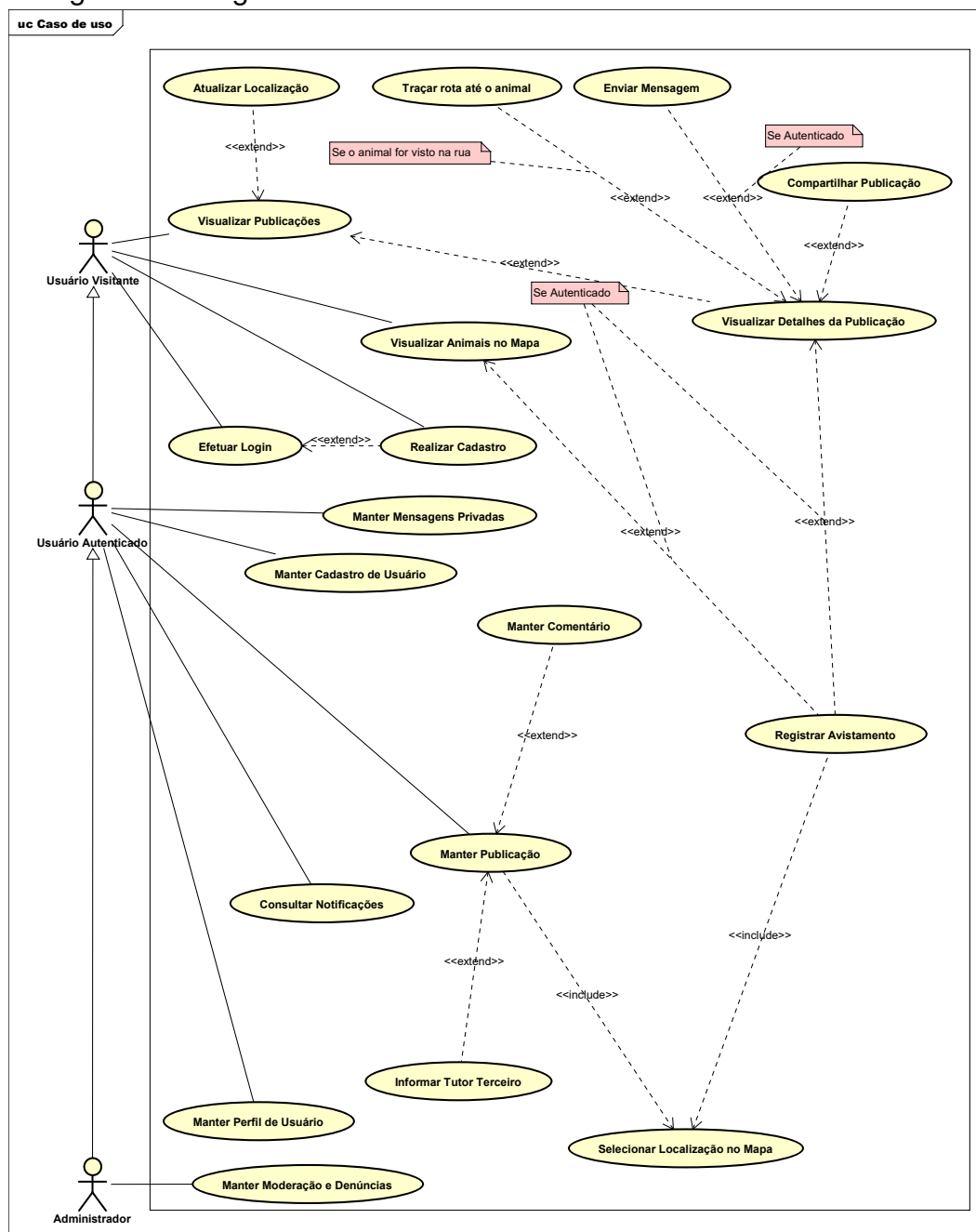
Figura 11: Diagrama de Casos de Uso Geral da Plataforma WeFIND
