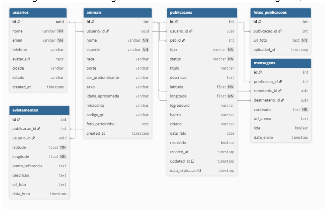
Figura 15: Modelo Lógico Relacional do Banco de Dados PostgreSQL
